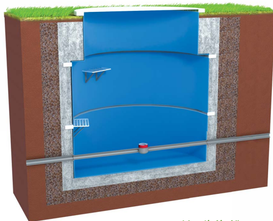
Vertikální řez vodoměrné šachty
